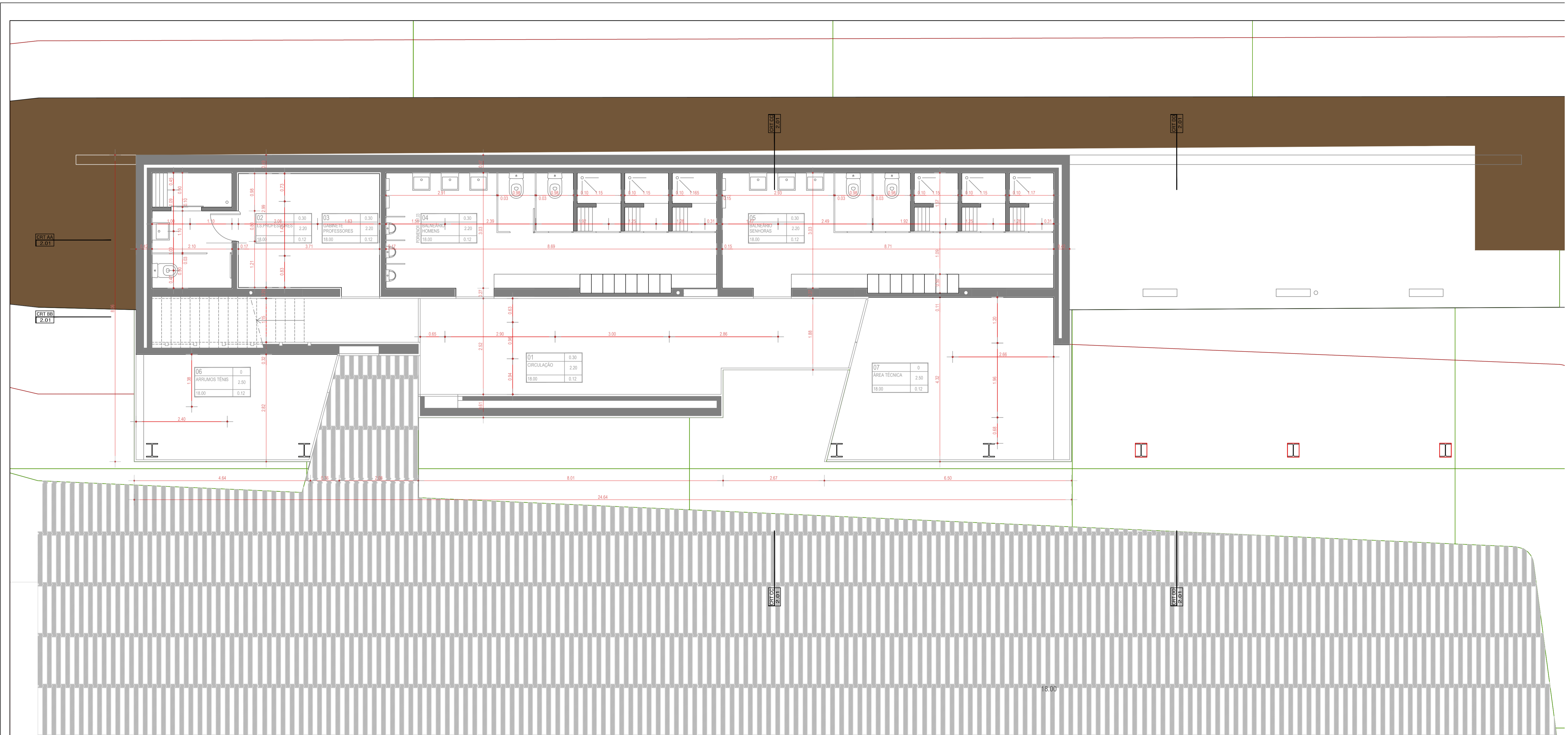
EDIFICIO DE APOIO AO CAMPO DE TÊNIS PLANTA DO PISO 0 ESC. 1/50
